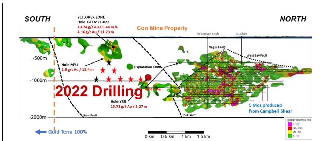
Abbildung 1 - Bohrprogramm 2022 auf Campbell Shear (Scherzone), Längsschnitt (Blick nach Westen)
