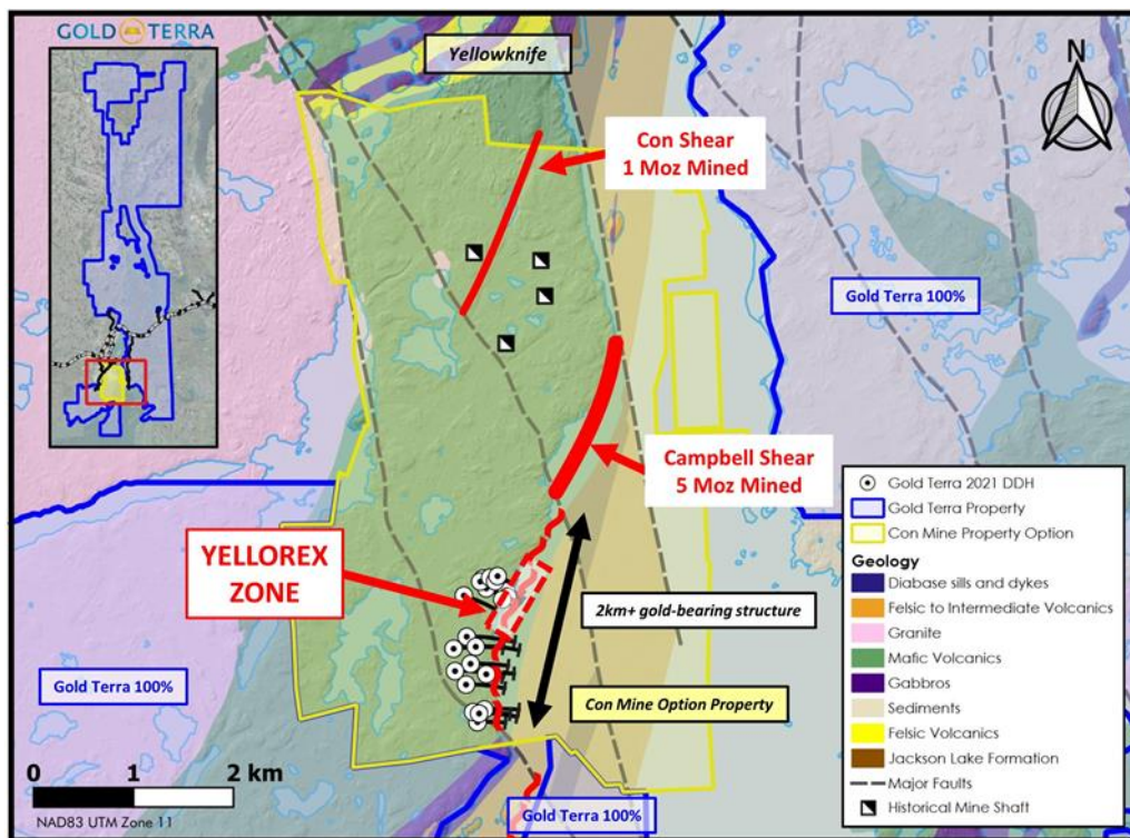
Abbildung 2 - Campbell-Scherzone
